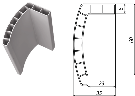
Наличник 60x35
