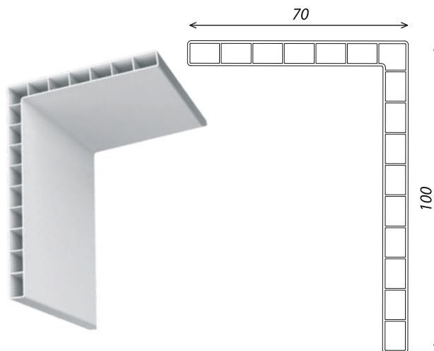
Наличник 70x100
