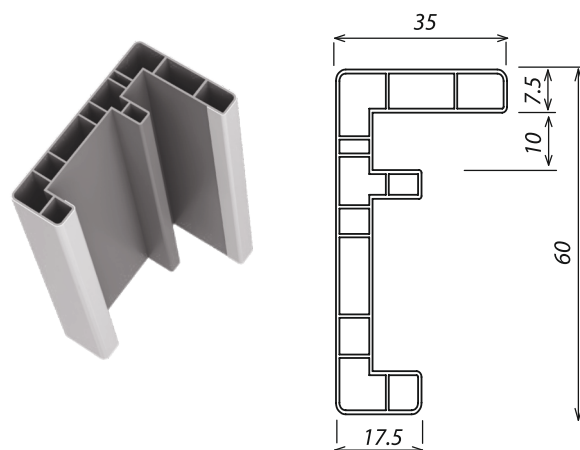
Наличник 60x35
